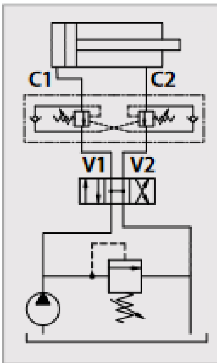
doppeltwirkend
