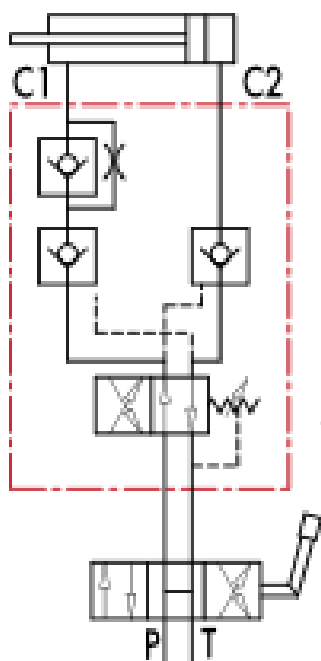
doppeltwirkend
