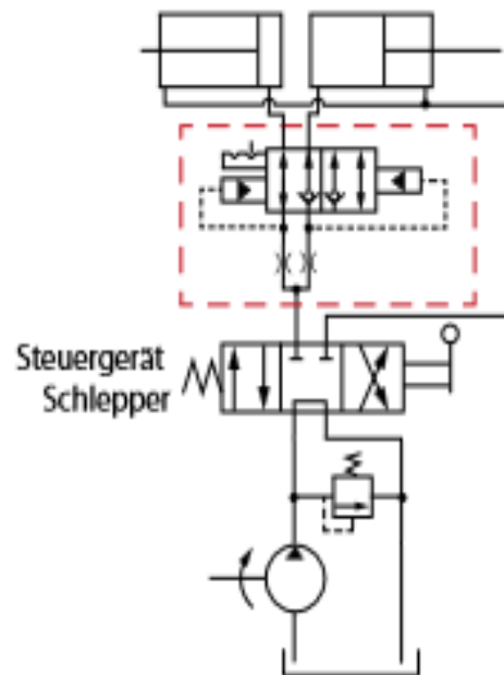
System mit doppeltwirkenden Zylindern
