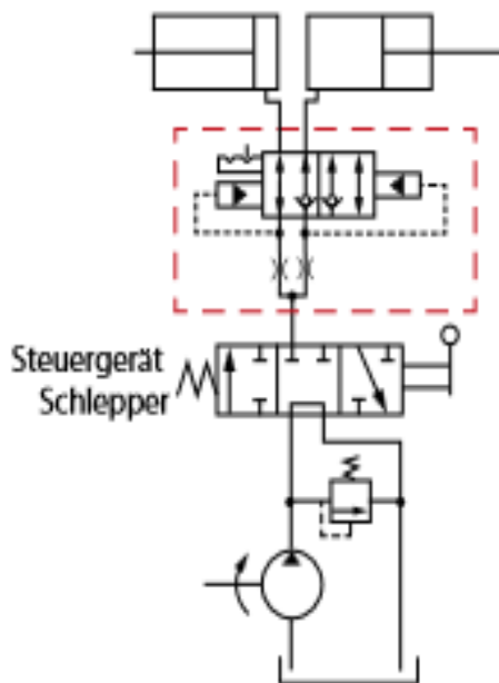
System mit einfachwirkenden Zylindern
