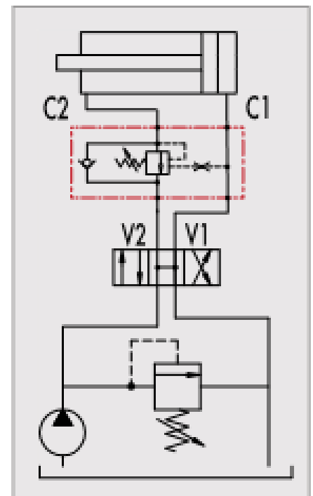
einfachwirkend
