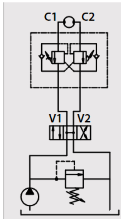
doppeltwirkend, OMP+OMR
